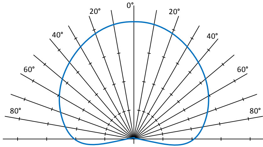
Рисунок 2.2 – Диаграмма направленности ДДЗ-01
