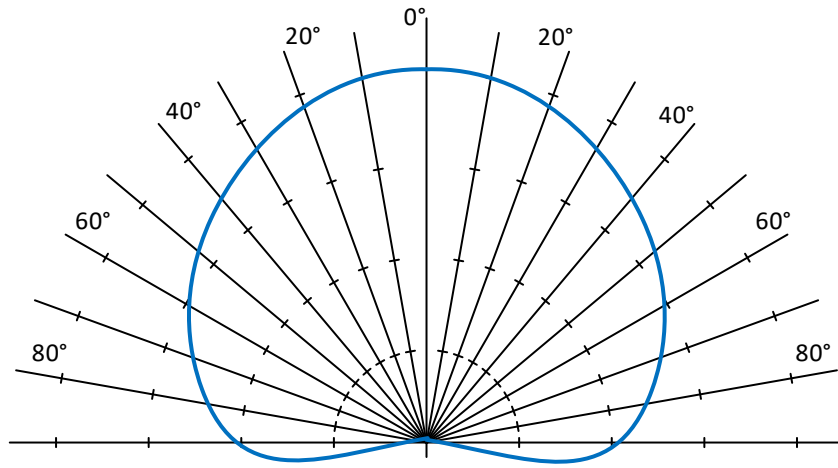
Рисунок 2.2 – Диаграмма направленности ДД3-01
