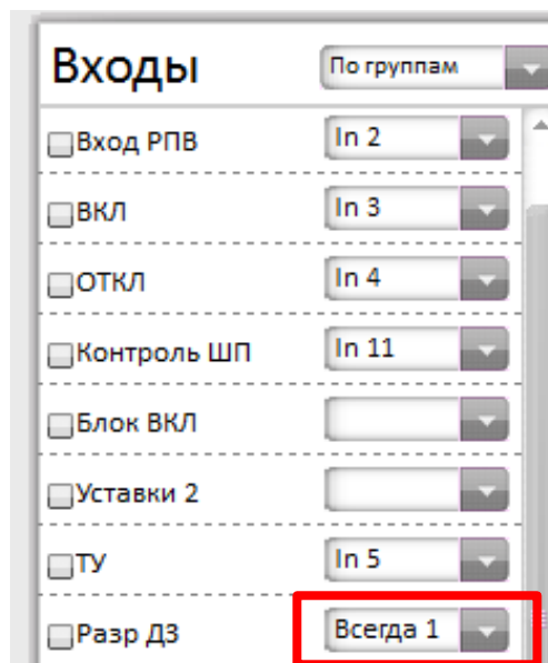
Рисунок 4.2 – Настройка защиты на примере устройства БЗП-03
