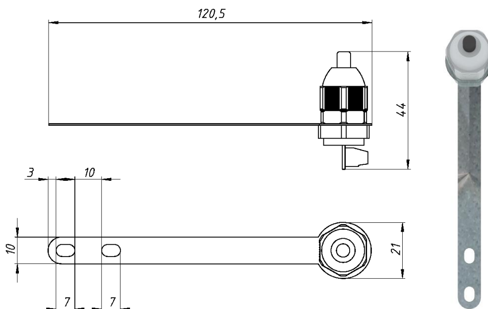
Рисунок 2.1 – Габаритные размеры датчика дуговой защиты
