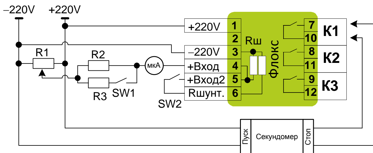
Рисунок 4.4 – Схема подключения для проверки реле Флокс
