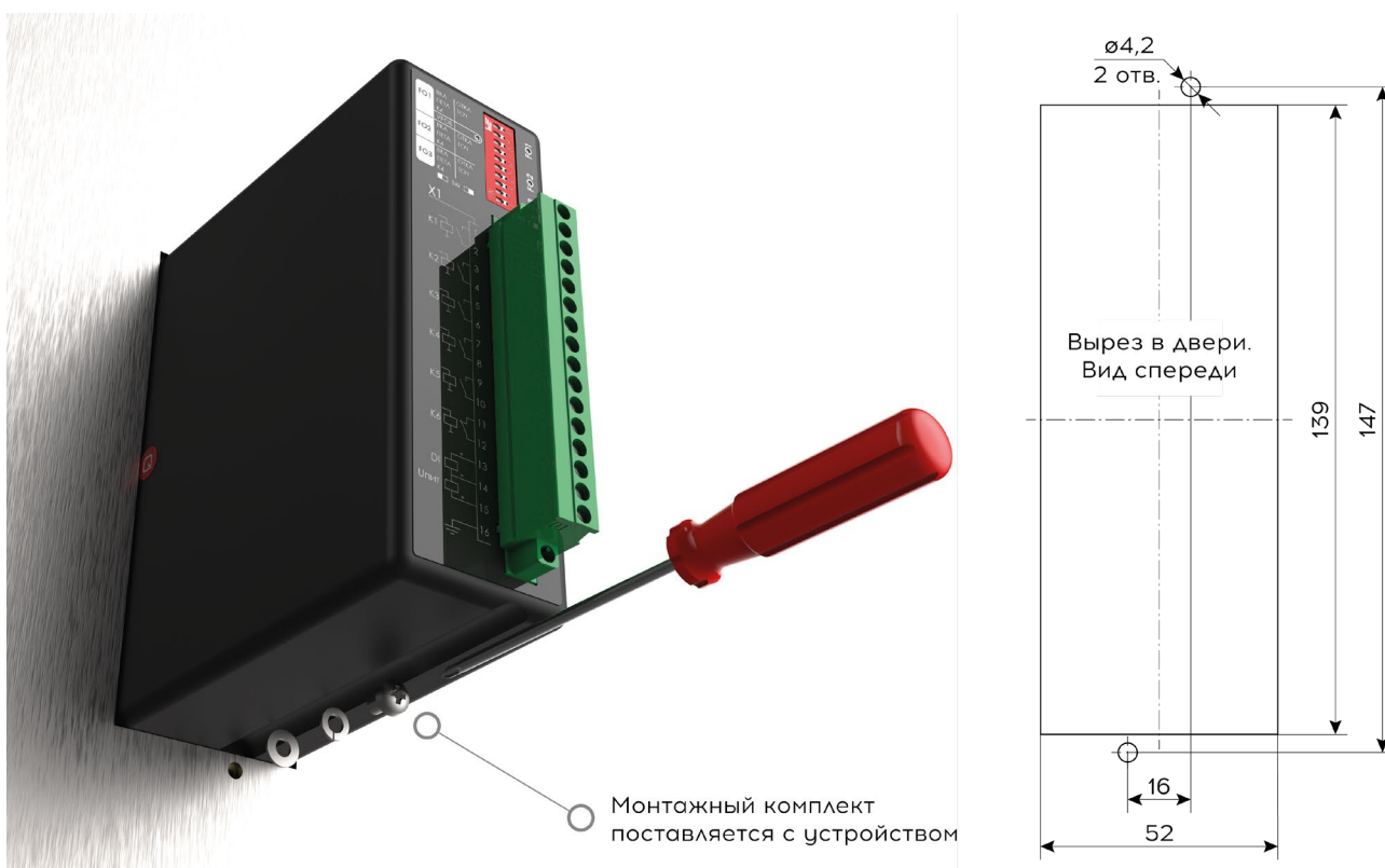
Рисунок А.10.2 – Установочные размеры на дверь
