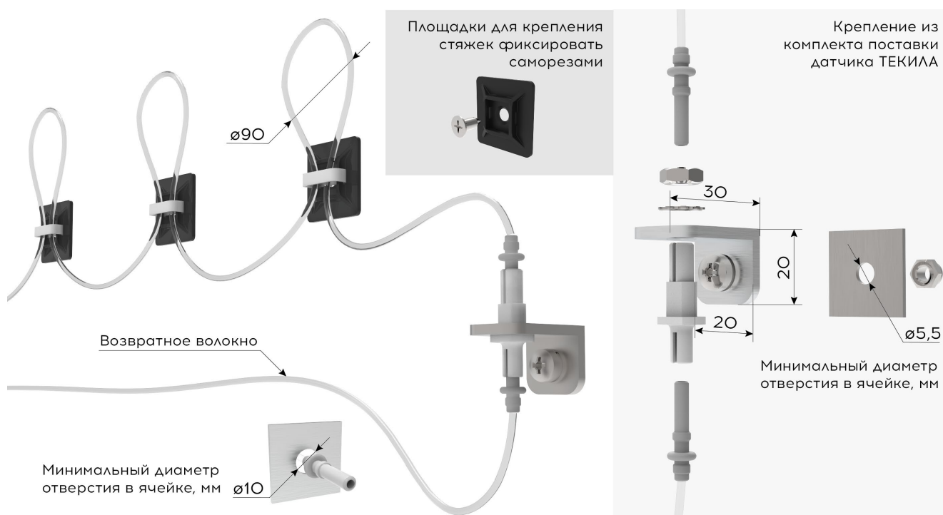
Рисунок 6.2 – монтаж петлевого датчика ТЕКИЛА
