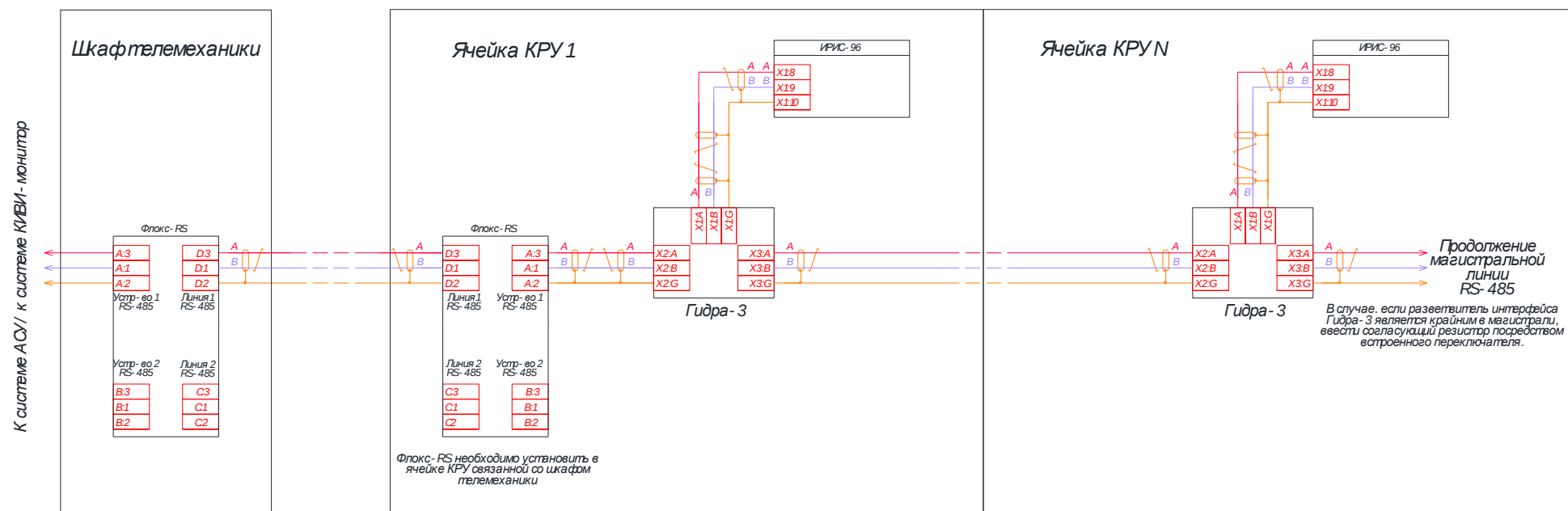
Рисунок 12.1 - Схема организации линий связи интерфейса RS-485 с применением устройств Гидра-3, Флокс-RS
