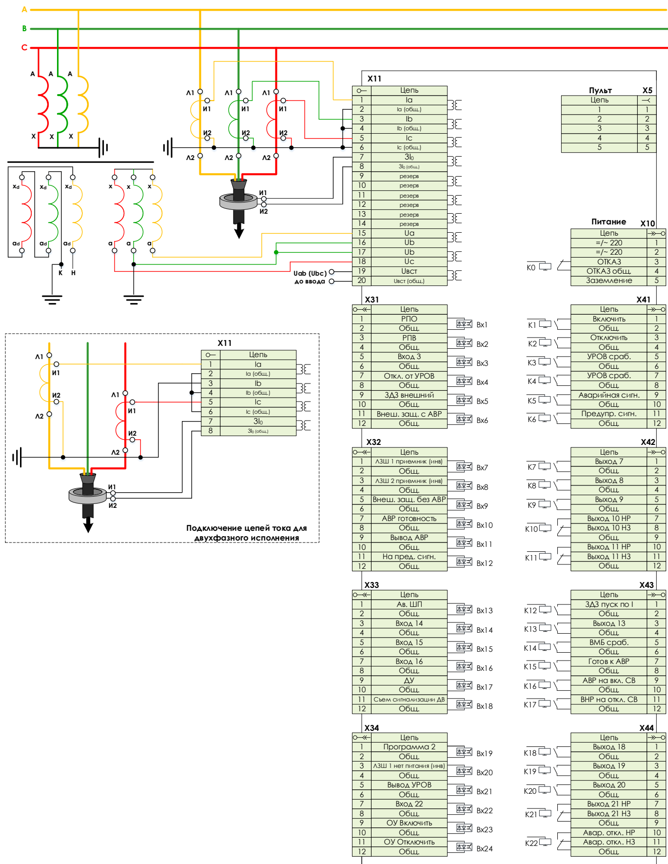
Рисунок 14.6 – Защита на вводном выключателе 6-10 кВ
