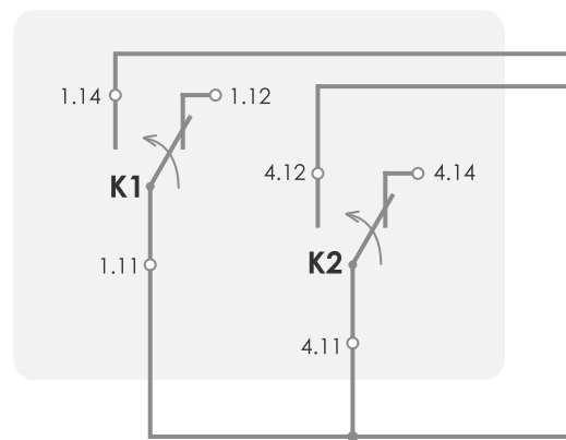
Рисунок 7.13 – Пример подключения вспомогательных контактов автоматического выключателя для контроля положения выключателя
