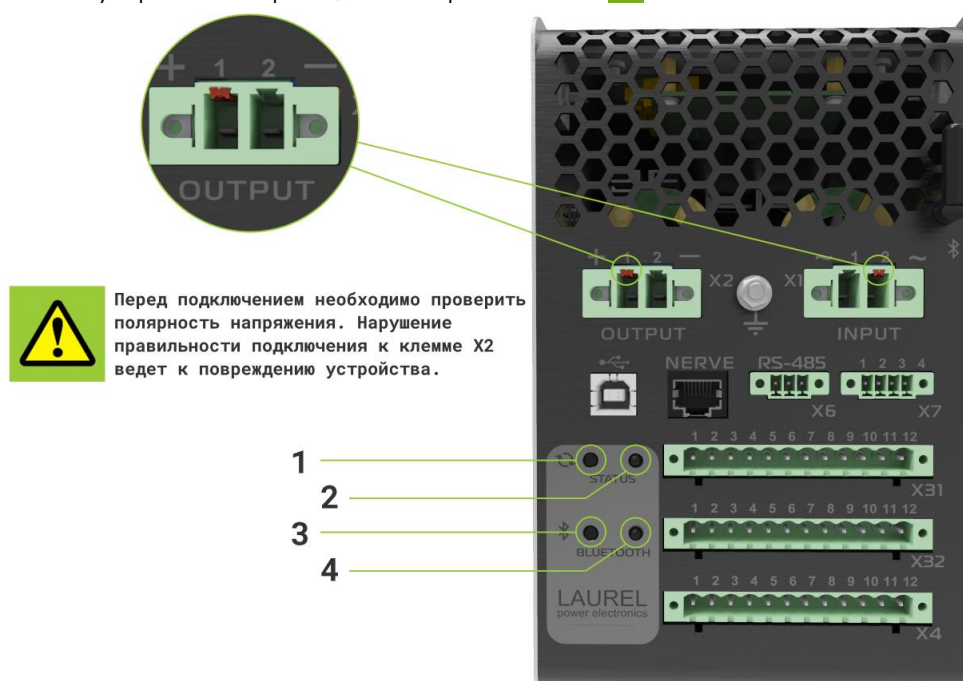
Рисунок 5.3 – Лицевая панель ЛАУРЕЛЬ
