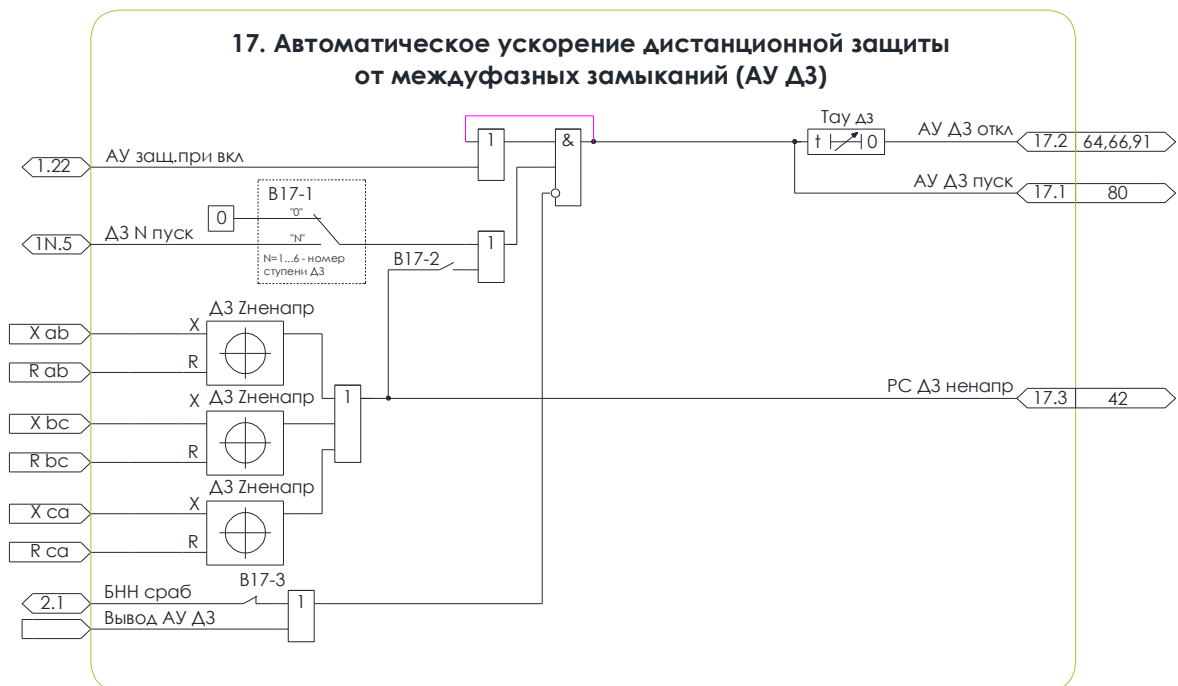
Рисунок 4.25 – Схема №17. Алгоритм автоматического ускорения ДЗ
