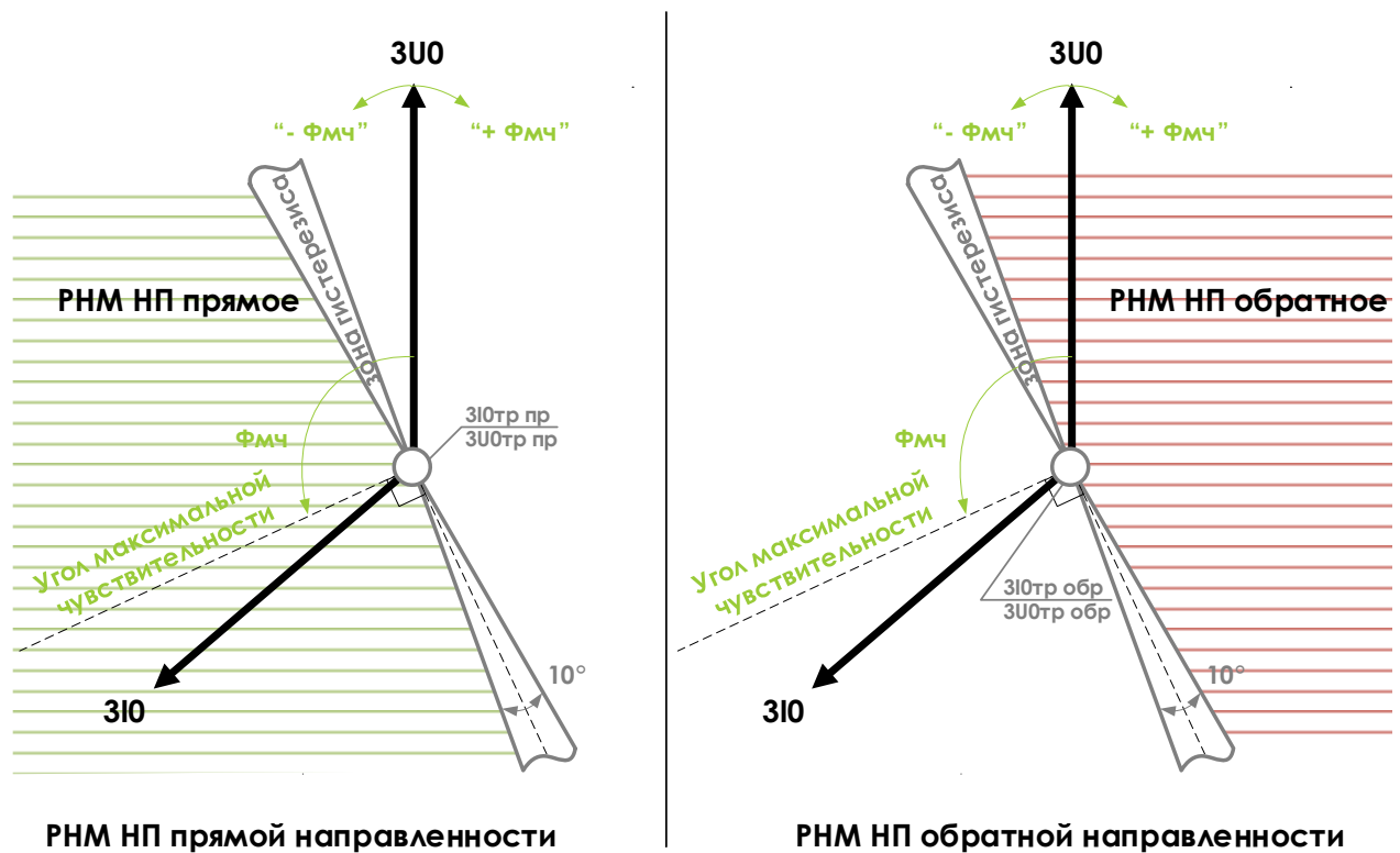
Рисунок 5.1 – Реле направления мощности нулевой последовательности
