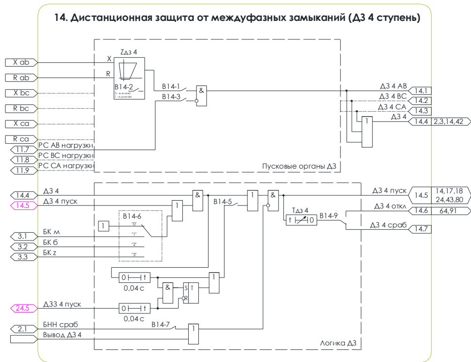
Рисунок 4.24 – Схема №14. Алгоритм четвертой ступени ДЗ
